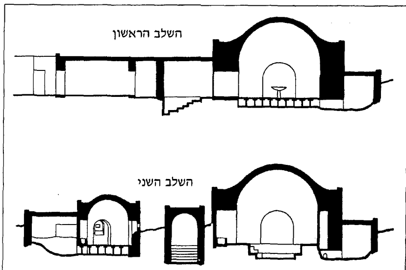
איור 3: חתך דרך בית-המרחץ בשלב הראשון ובשלב השני
