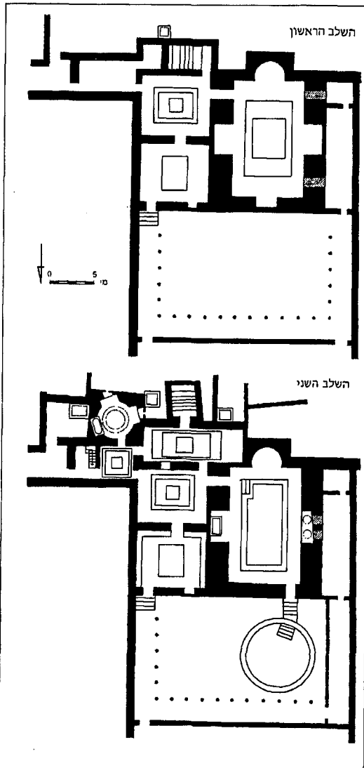
איור 2: תכנית בית-המרחץ בשלב הראשון ובשלב השני
